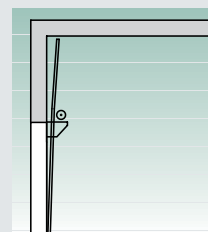
Kování WB Svislé kování s dole umístěnou hřídelí s torzními pružinami
