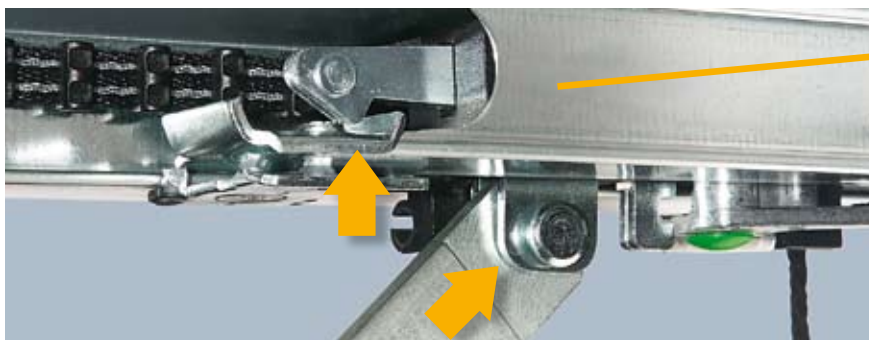
Uzavření vrat v kolejnici pohonu - patent společnosti Hörmann
